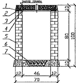
РАЗРЕЗ А-А
