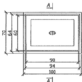
ДЕТАЙЛ - ШАХТА 60/90
